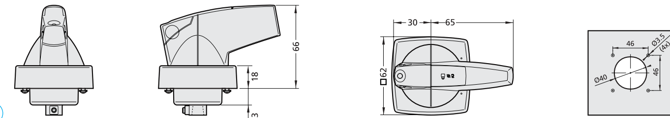
Type K2D en K2SD
